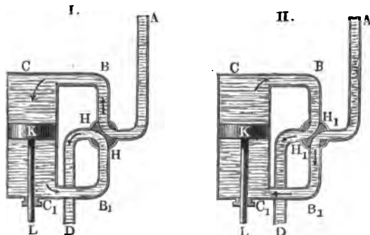
Fig. 11 und 12. Wasserfäulenmaschine.
